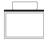
60cm Wall Hung Single Unit 600(w) x 402(h) x 455(d)mm (Excl. Basin) One soft close drawer
