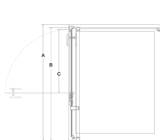
Frameless hinged door
